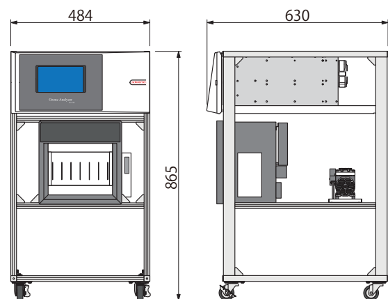
ラック組込型 (A0865) (約35kg, ポンプ重量を含む)
